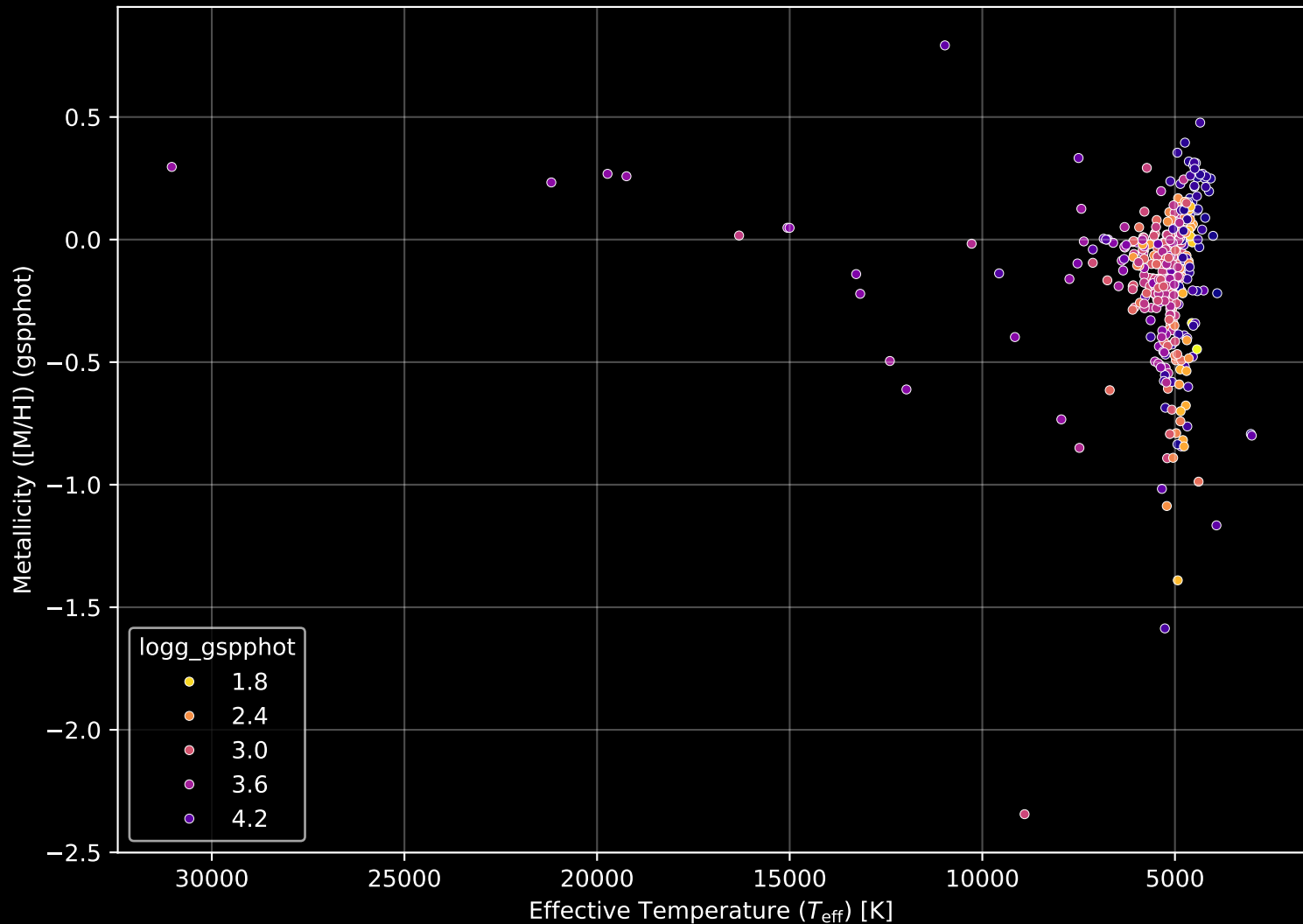
APOGEE DR17 Field: [180+04] Stellar Population Parameters (n= 431)
